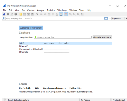
Fig. 3.14. Herramienta Wireshark.
