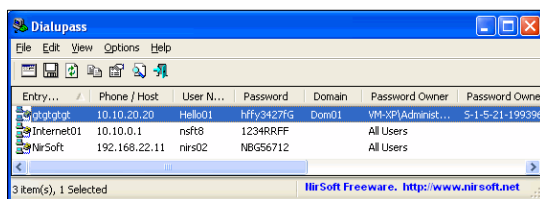
Fig. 2.33. Artefacto Dialupass.
