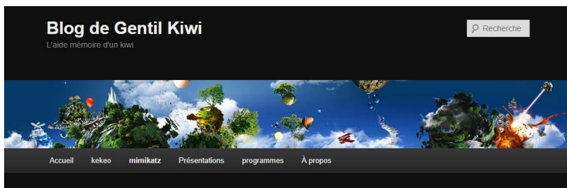
Fig. 3.12. Mimikatz.
